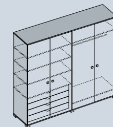
333 L H.2140 L.2400 S.600 H.2340* 359/374* кг - 0,92/0,94* м³
