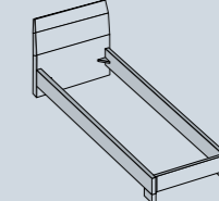
341/1 H.930 L.2200 S.900 67 кг - 0,3 м³
