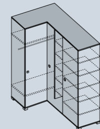
335 R H.2140 L.1800 S.1200 H.2340* 310 кг - 0,9 м³
