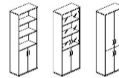
Шкаф высокий широкий A.ST-1.1 770x365x1980 мм A.ST-1.2 770x365x1980 мм A.ST-1.3 770x365x1980 мм
