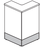
Угловой модуль левый/правый Л.УМ-1 Л/Пр 736x736x1156 мм
